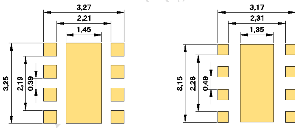
建议焊盘图
