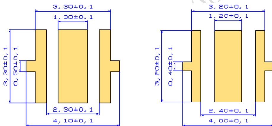
建议 PCB 焊盘
