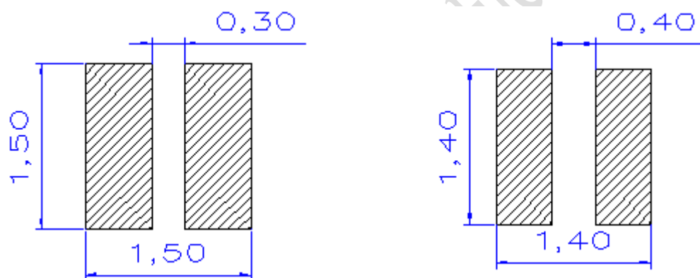
建议 PCB 焊盘
