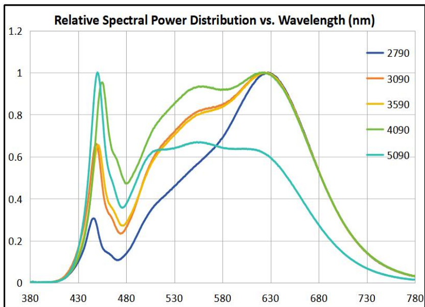
Fig 1. 相对光谱分布特性 Relative Spectrum Distribution Characteristics
