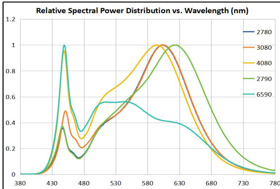
Fig 1. 相对光谱分布特性 Relative Spectrum Distribution Characteristics
