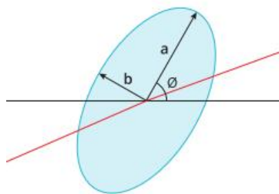
关于 3 步、5 步麦克亚当椭圆的说明 3- and 5-step MacAdam ellipse illustration
