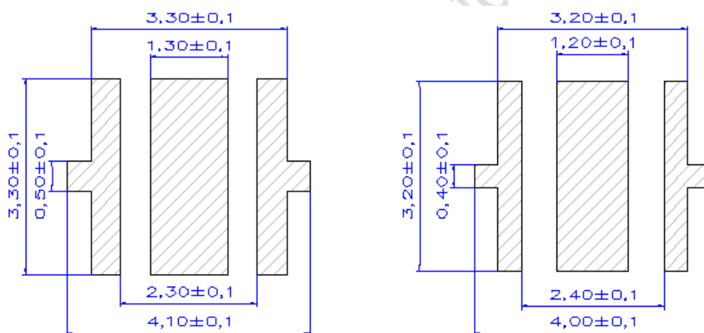
建议 PCB 焊盘
